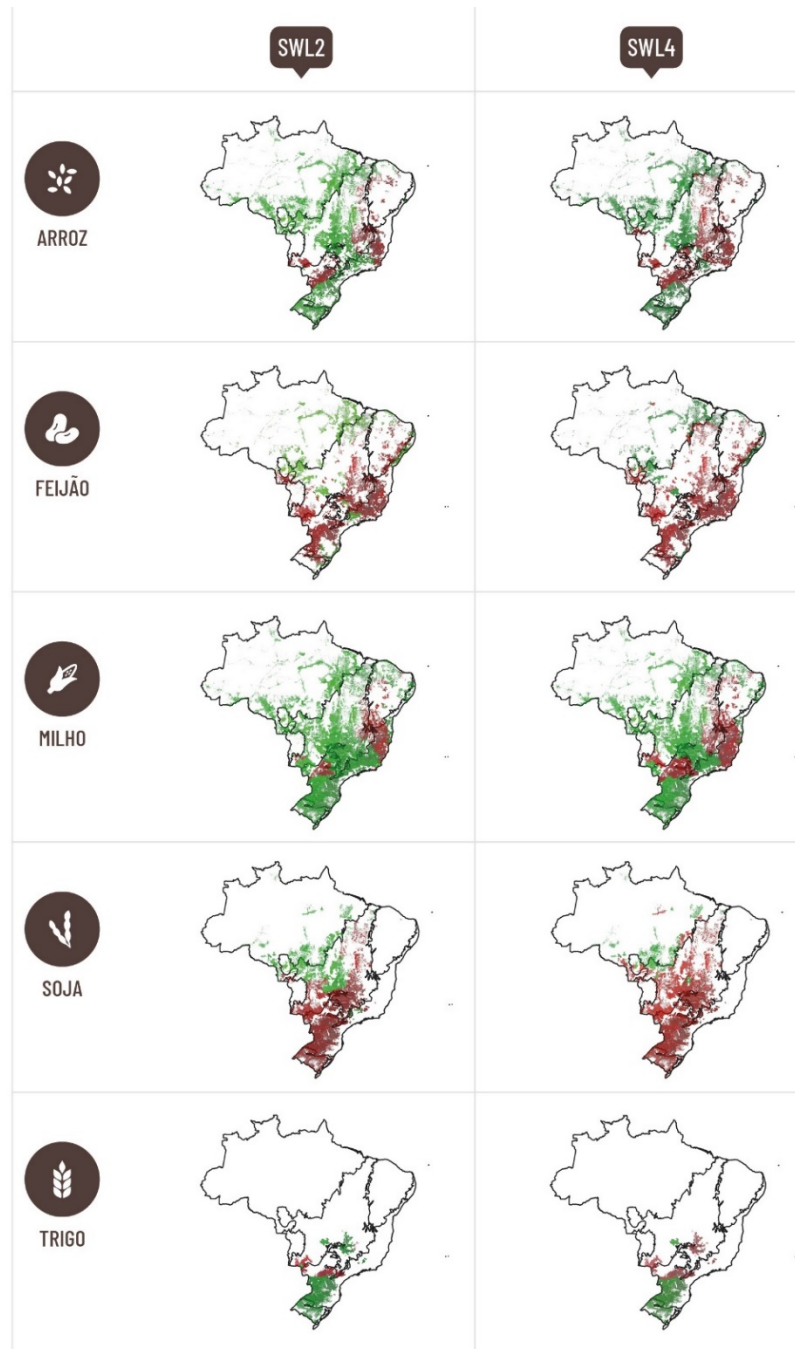
Figura 3.37. Zoneamento Agrícola de Risco Climático (ZARC) para as principais culturas agrícolas que compõem a segurança alimentar no Brasil, considerando os SWL2 e SWL4 (período futuro). Fonte: MCTI (2016).
