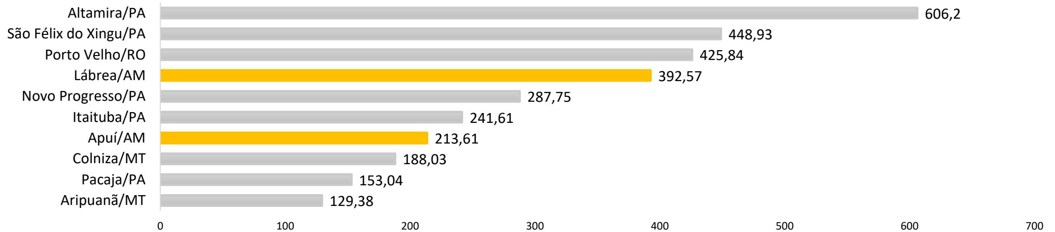
Figura 01: Ranking dos Estados e Municípios da AMZ (01/jan - 16/out). Fonte: Terrabrasilis – INPE
