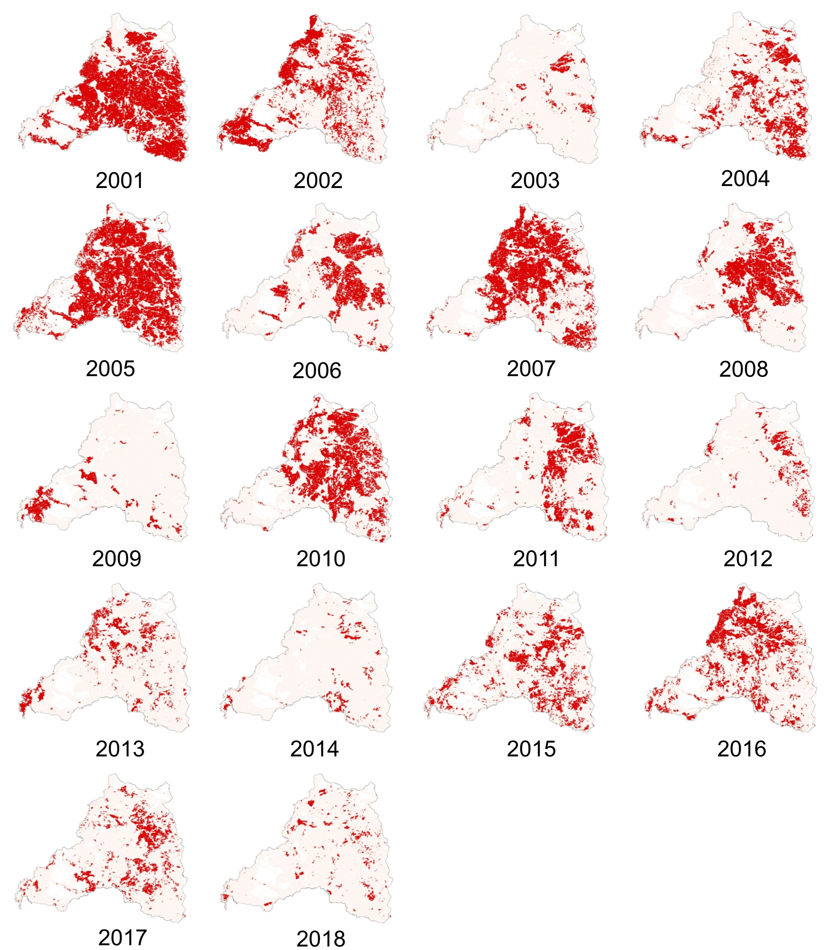
Figura 2 – Cicatrizes de queimadas, representadas pela cor vermelha, mapeadas para a terra indígena Kadiwéu ano a ano, no período de 2001 a 2018.
