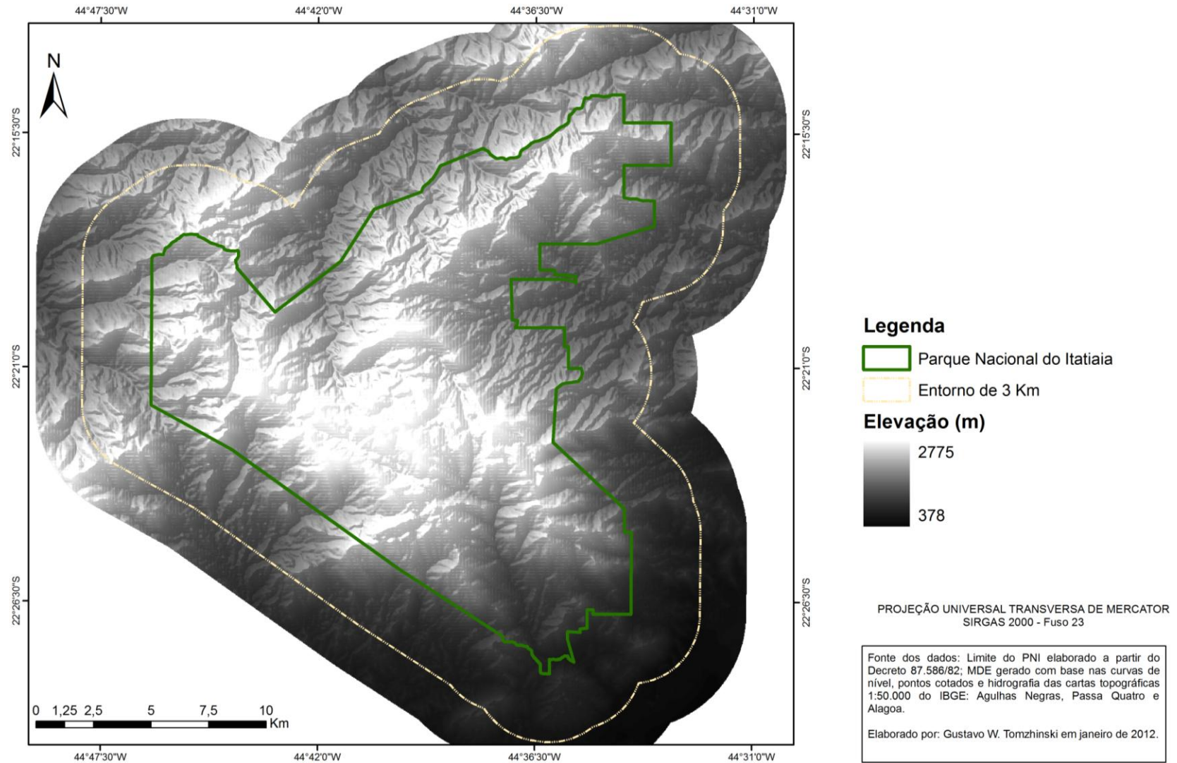
Figura 29 – Modelo Digital de Elevação gerado para a Área de Estudo
