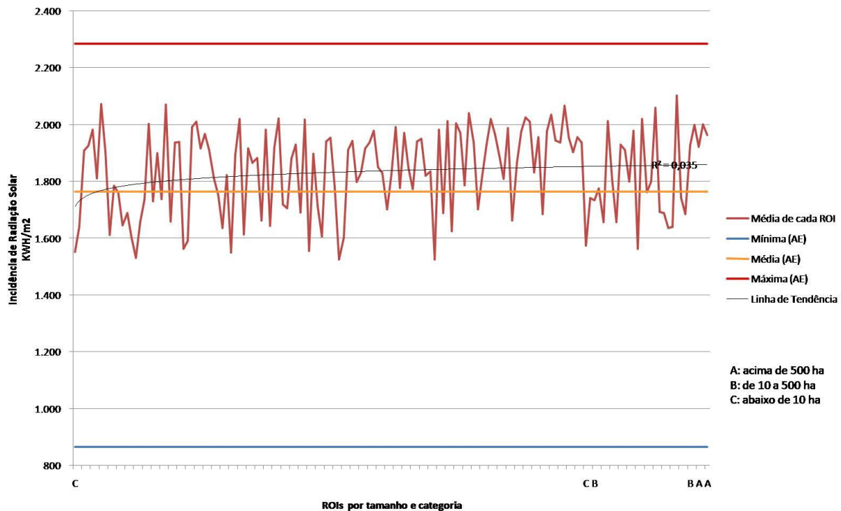
Figura 31 – Incidência média de radiação solar para os polígonos de incêndios estudados em comparação com os valores máximo, mínimo e médio encontrados para toda a Área de Estudo (AE).
