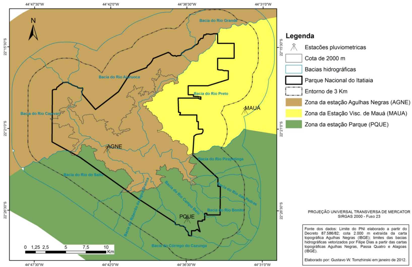
Figura 47 – Mapa de localização das estações pluviométricas com as respectivas zonas de abrangência estimadas
