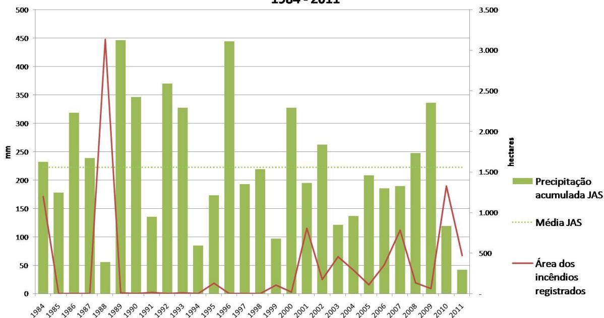
Figura 50 – Gráfico comparativo do acumulado trimestral de precipitação julho-agosto-setembro (JAS) para o período de 1984 a 2011 com os as áreas dos registros históricos de incêndios.
