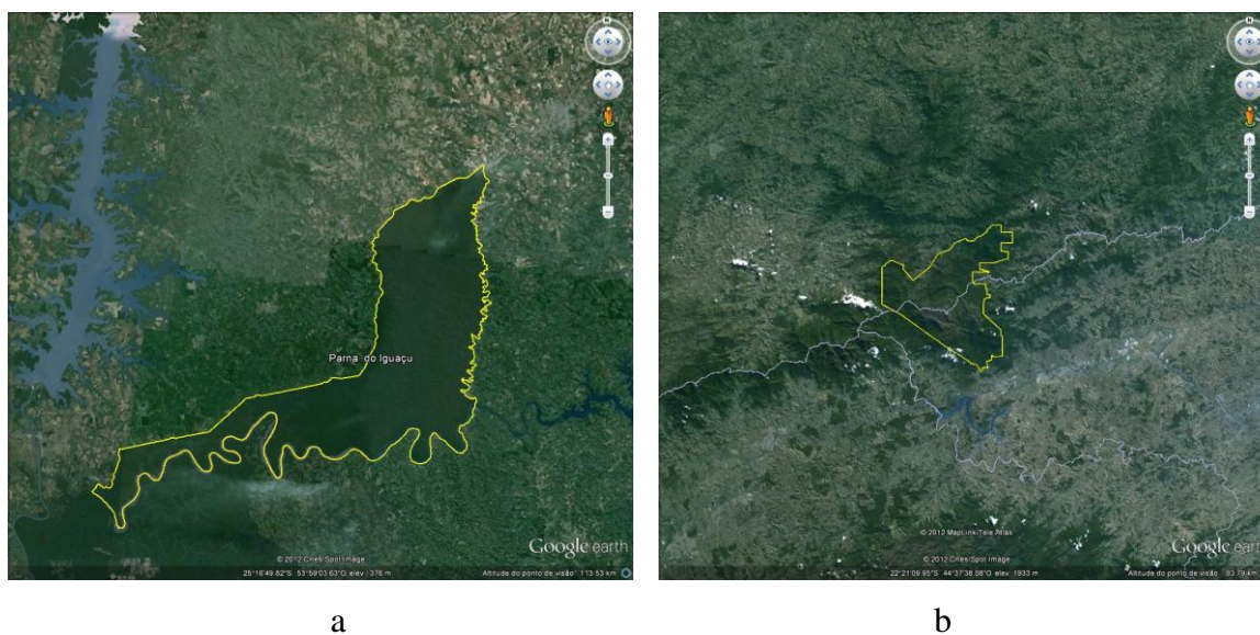
Figura 4 – Imagens do Google Earth™ dos Parques Nacionais do Iguazu (a) e Itatiaia (b). Acesso em 21/02/2012.
