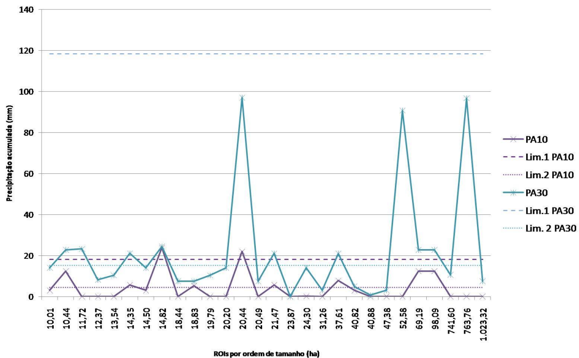
Figura 55 – Gráfico da relação entre PA10 e PA30 e os ROIs maiores que 10 ha.
