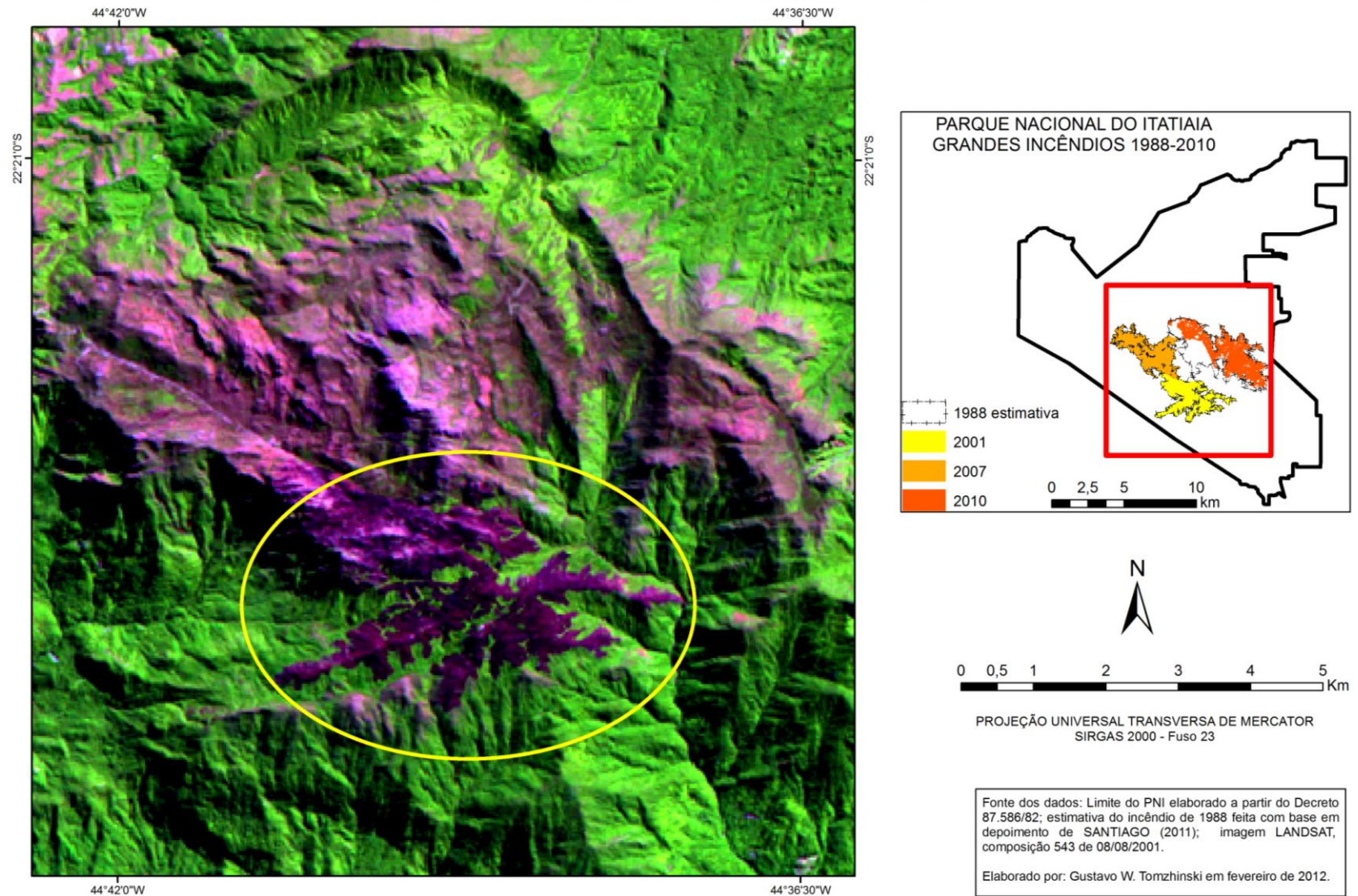
Figura 16 – Carta Imagem do Incêndio no Planalto de 2001, com destaque para a área queimada dentro da elipse amarela.
