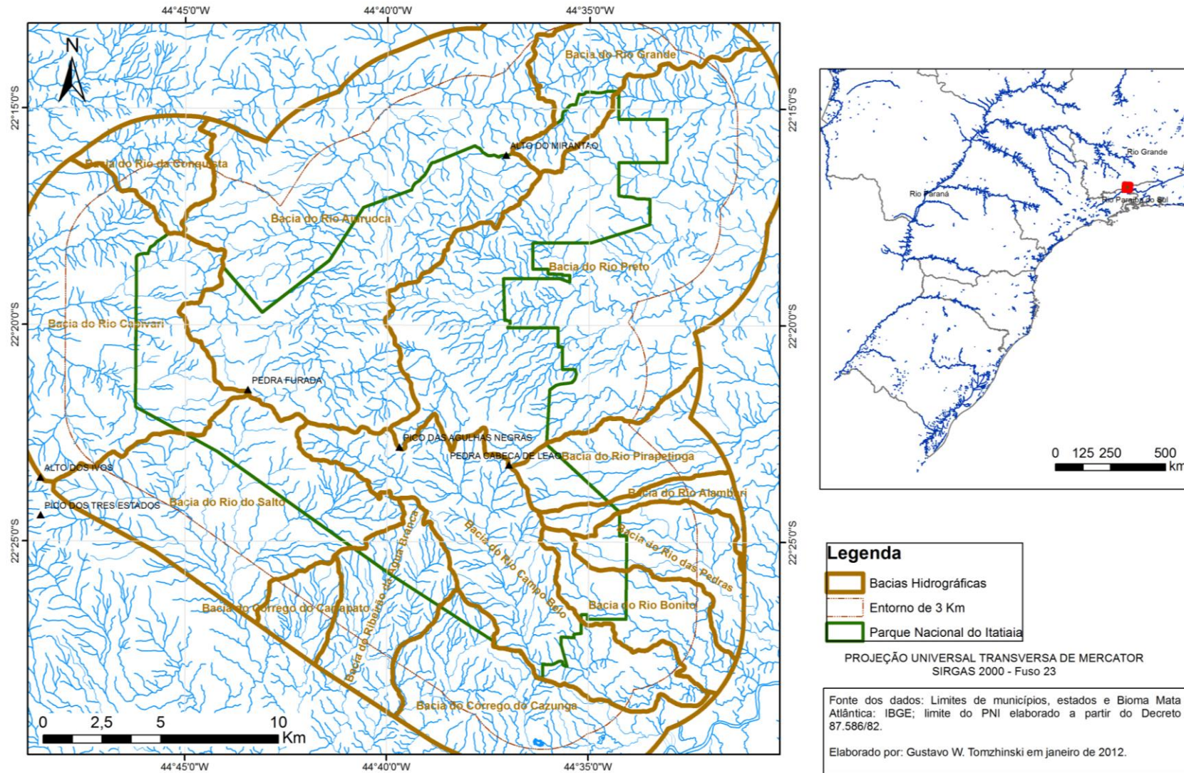
Figura 9 – Hidrografia da Área de Estudo (AE), incluindo as principais bacias hidrográficas.
