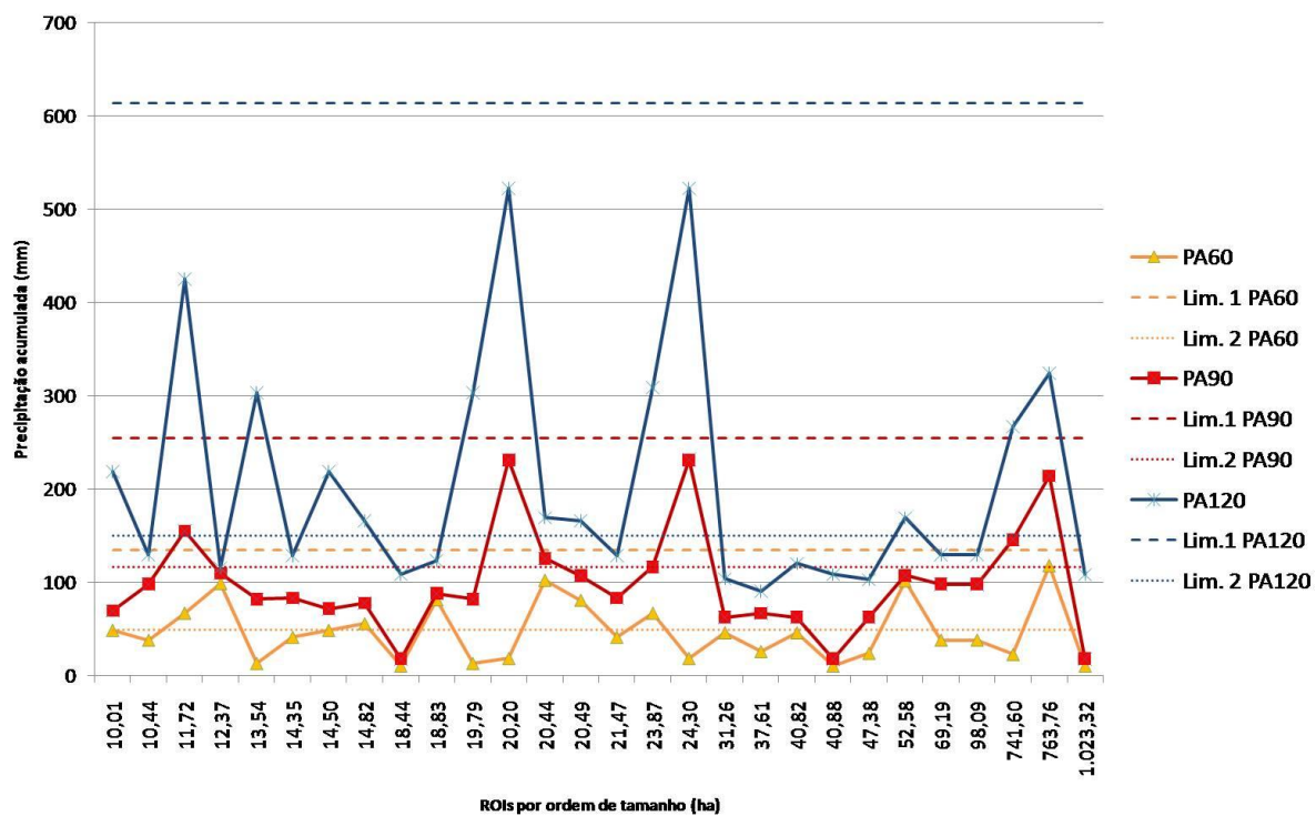
Figura 56 – Gráfico da relação dos indicadores de médio prazo com os ROIs maiores que 10 ha.
