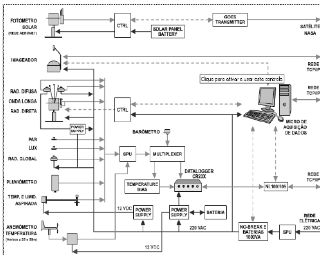
Figura 6.3 – Diagrama da configuração local dos equipamentos instalados na Estação SONDA – SMS no Observatório Espacial do Sul – OES/CRS/CIE/INPE – MCT. Fonte: SONDA (2007).
