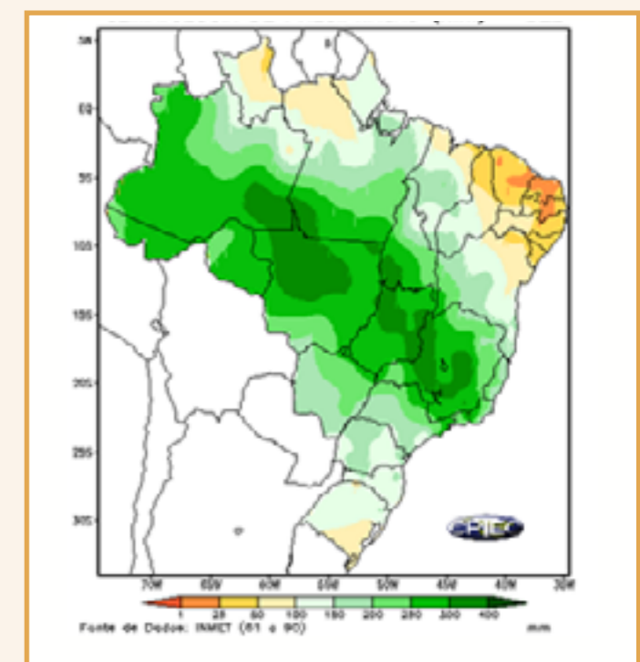
Mapa 2.2: Climatologia de Precipitação (mm) Dezembro
