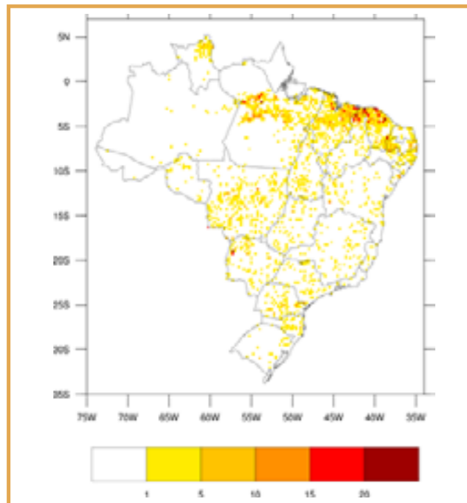
Mapa 1.1: Total de detecções registradas em Dezembro/2018
