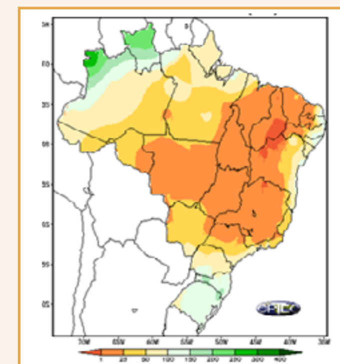
Mapa 2.2: Climatologia de Precipitação (mm) Agosto
